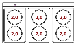
PŘÍKON PLOTÝNEK
