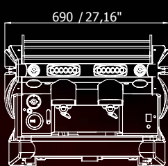
Boiler: lt.6 / lt.8 - 2gr. compatta
