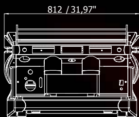
Boiler: lt.14 / lt.14 - 2gr.
